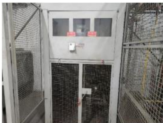
Figura 49 – Cabine da concessionária instalada no interior da SE.
